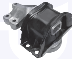
SUPPORTO motore (anteriore - dx) 2.0 HDi
